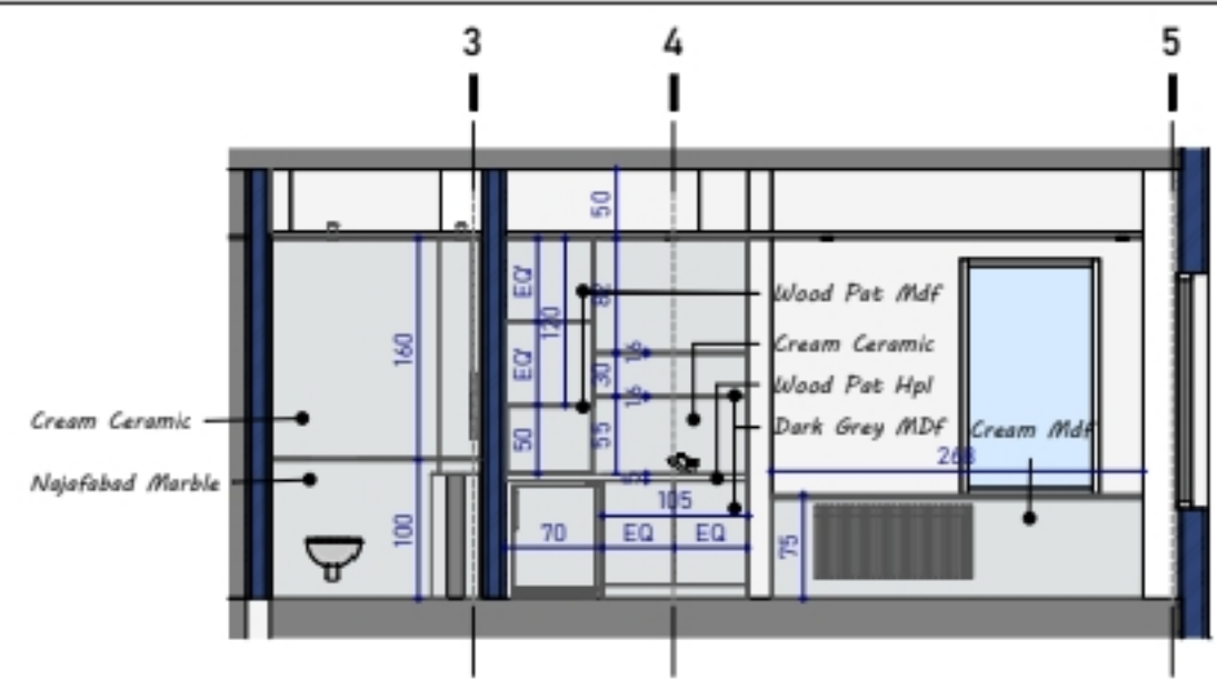
2. SECTION 39 1 : 50
