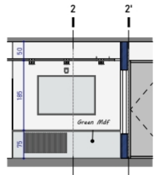
4. SECTION 51 1 : 50
