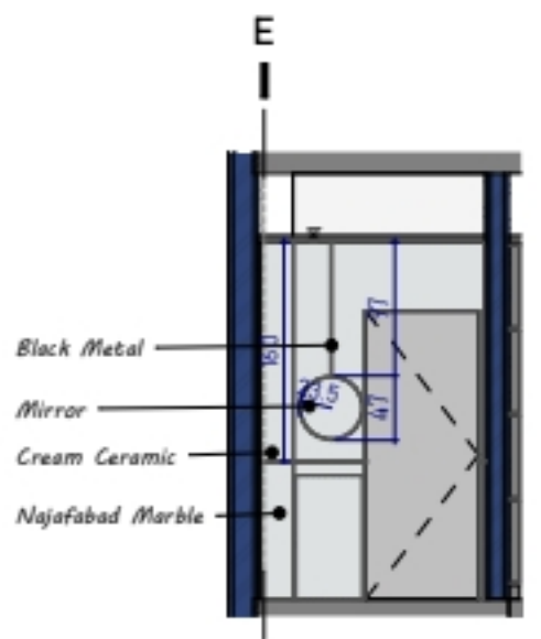
2. SECTION 39 1 : 50
