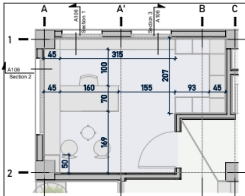
1. G.F - Layout 01
