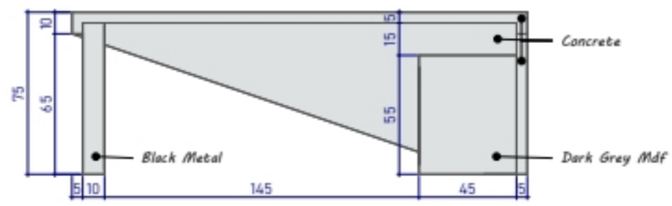
3. O-O 1 : 20
