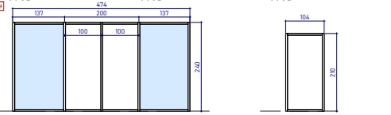
8. Door 03 1 : 50 9. Door 04 1 : 50
