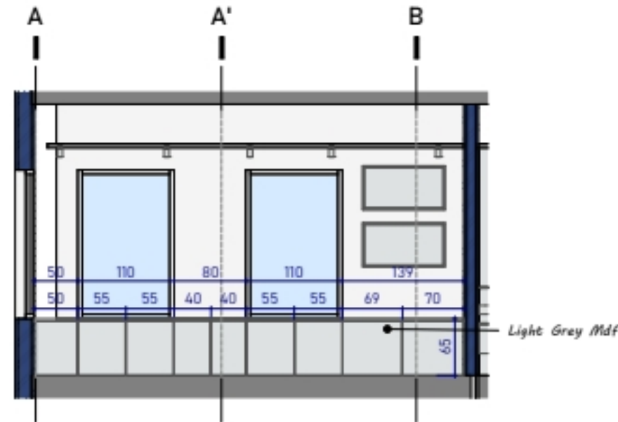
3. SECTION 50 1 : 50
