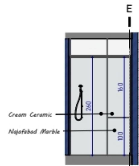
4. SECTION 41 1 : 50
