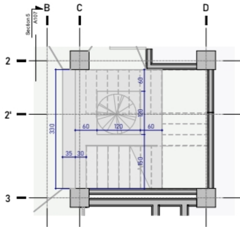
1. G.F - Layout 02
