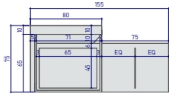
4. P-P 1 : 20
