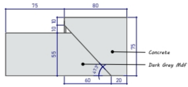
2. N-N 1 : 20
