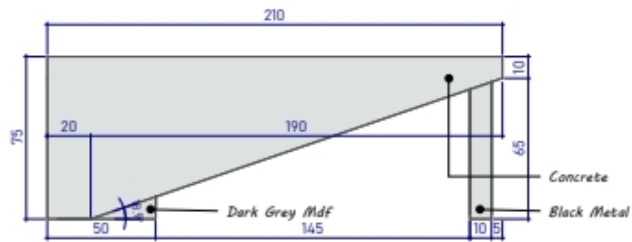
1. M-M 1 : 20
