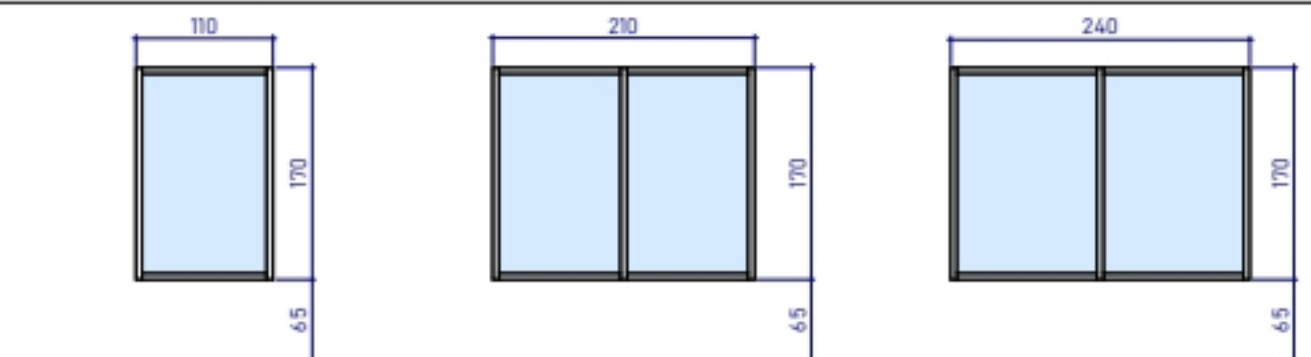
2. Window 01 1 : 50 3. Window 02 1 : 50 4. Window 03 1 : 50
