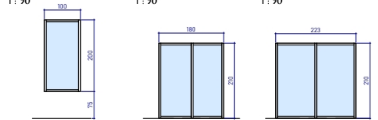
5. Window 04 1 : 50 6. Door 01 1 : 50 7. Door 02 1 : 50
