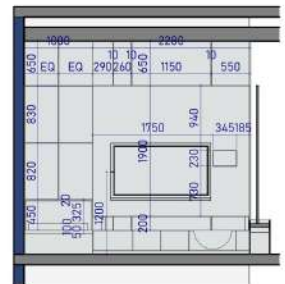
6. SECTION 4 1 : 50
