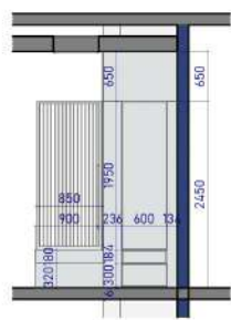
2. SECTION 1 1 : 50
