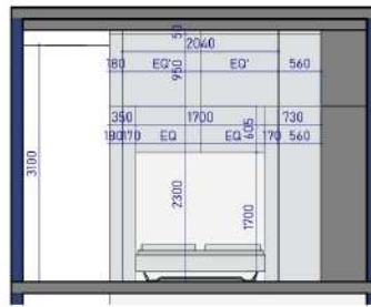
3. SECTION 11 1 : 50
