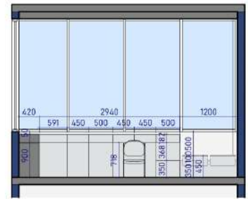
7. SECTION B 1 : 50
