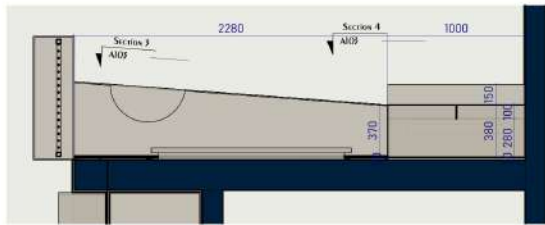
4. Tv Wall Layout 1 : 25
